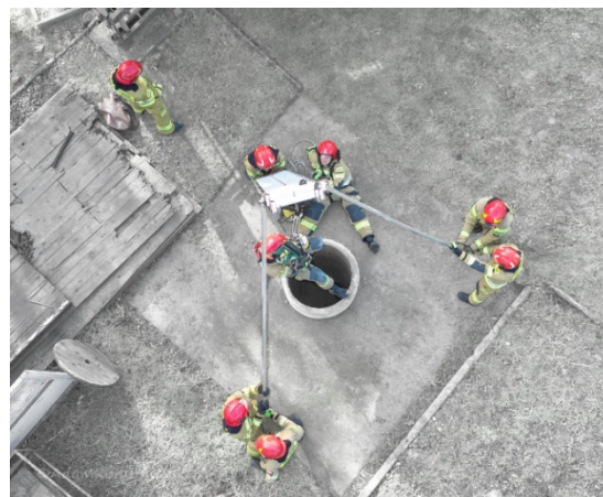
Drabina wolno stojąca (układ 4:1 do studni)
